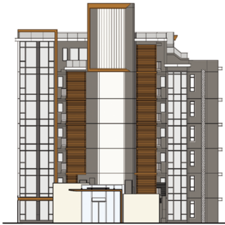
ELEVATION 2 立面圖 2
