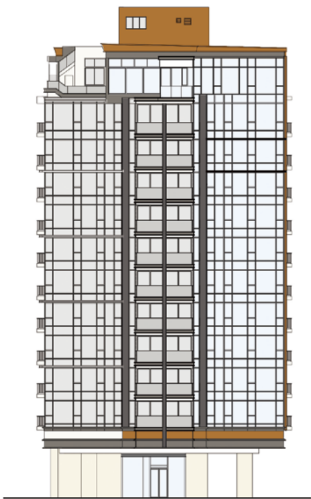
ELEVATION 4 立面圖 4
