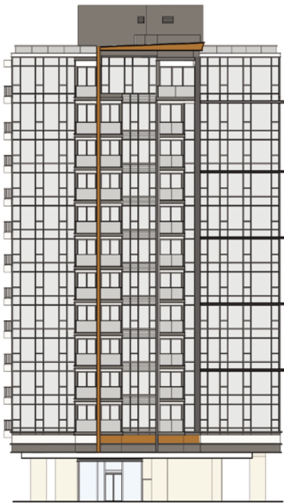
ELEVATION 3 立面圖 3
