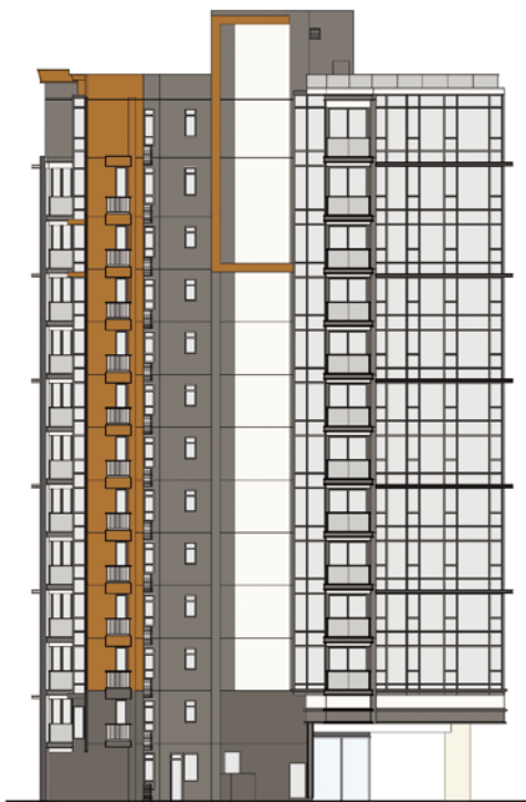
ELEVATION 5 立面圖 5
