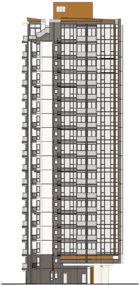
ELEVATION 4 立面圖 4
